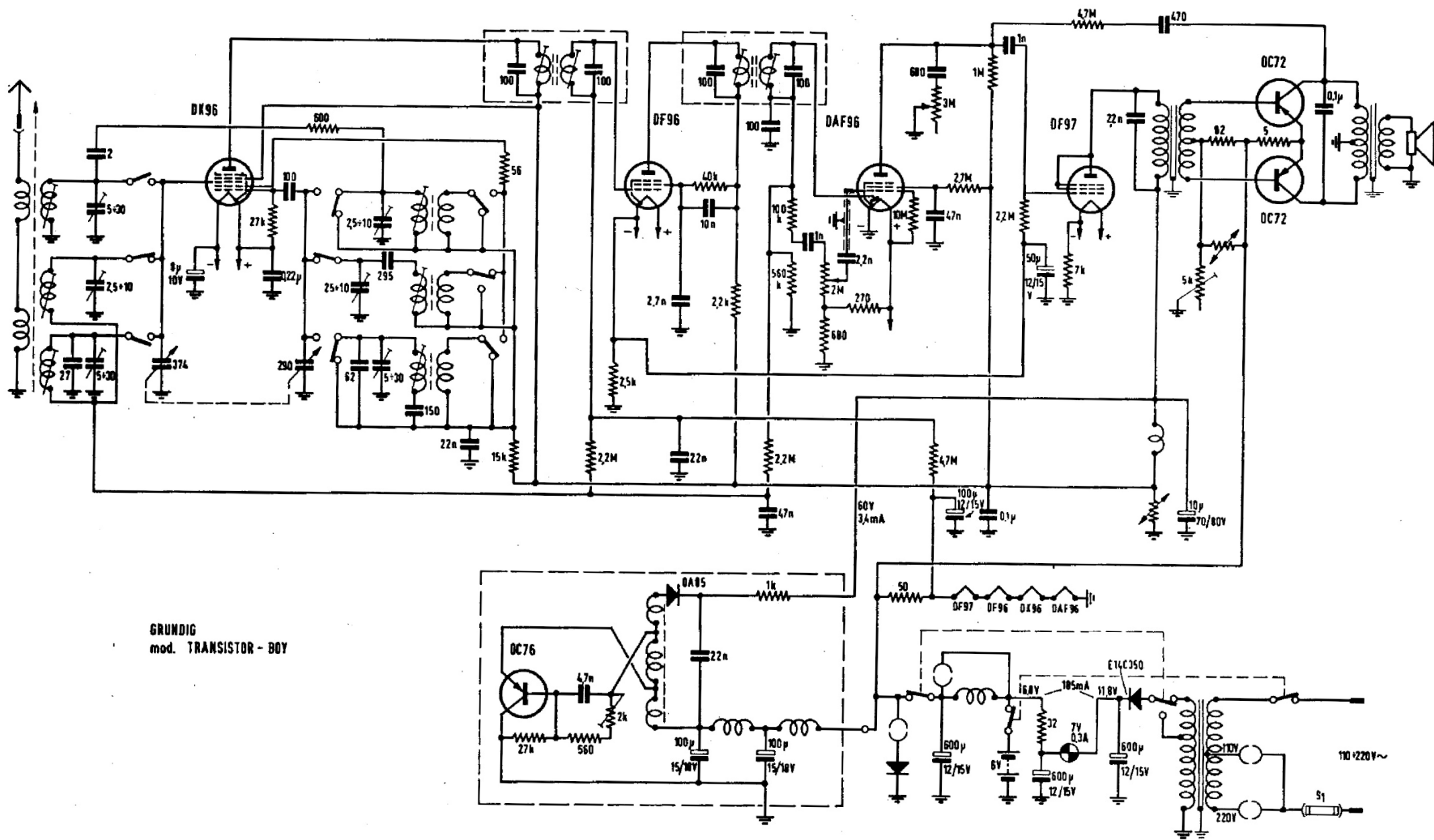
SCHEMA ELETTRICO DEL RADIORICEVITORE AM GRUNDING, MOD. TRANSISTOR BOY
